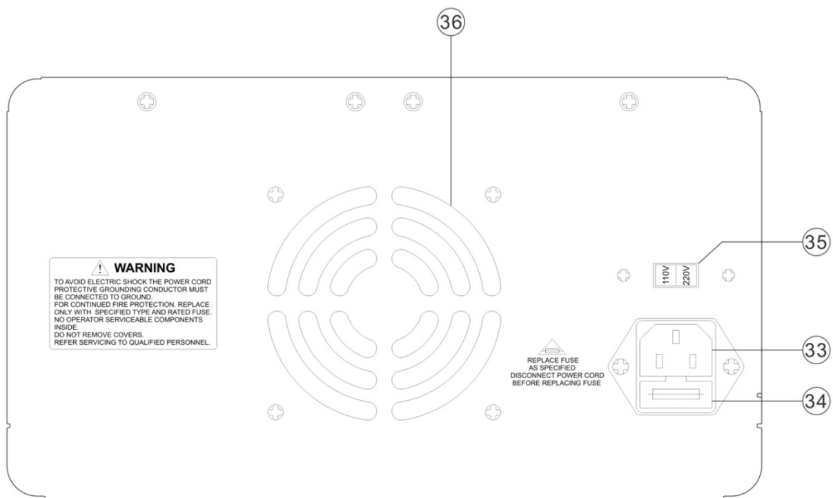
圖 3.2 後面板
