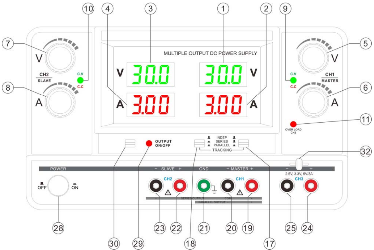
圖 3-1 前面板
